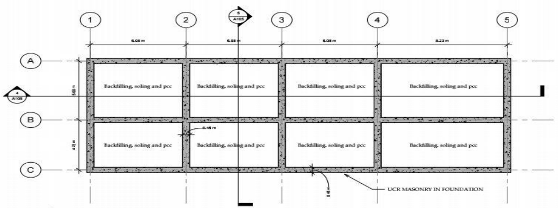
② GL 1 : 100
