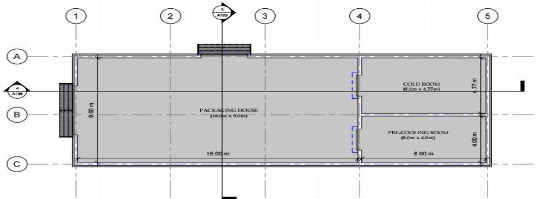
① Level 1 1 : 100
